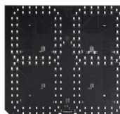
Art.0430-2520 ...F1502 scheda LED per INOUT-2s con 2 cifre Rosse + 2 cifre verdi Peso: 0,173kg.
