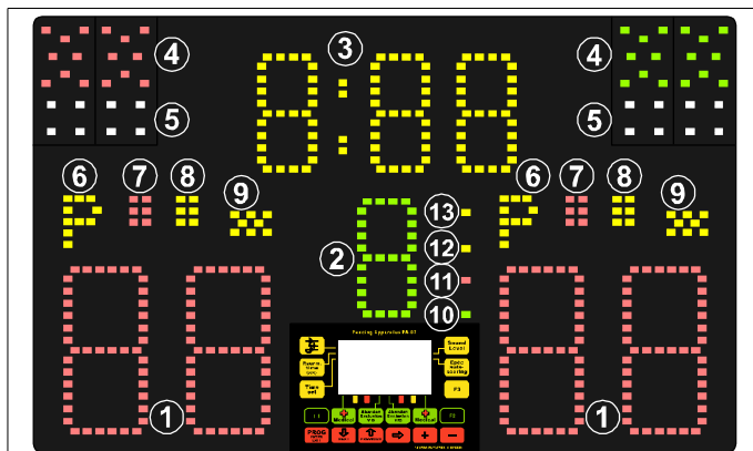
Fig. 1: Indicaciones luminosas mediante LEDs
