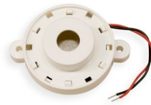
Art.0048-0160 Zumbador (buzzer), 105db-30cm Pieza de recambio Dimensiones: 4.5x6x3cm. - Peso: 0.02kg.
