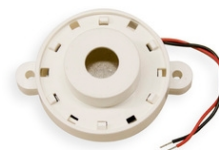
Art.0048-0160 Zumbador (buzzer), 105db-30cm Pieza de recambio Dimensiones: 4.5x6x3cm. - Peso: 0.02kg.
