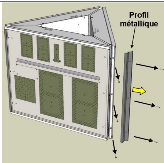
Fig. 15: Démontage des profils métalliques latéraux
