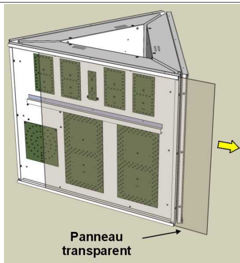
Fig. 16: Retrait du panneau frontal
