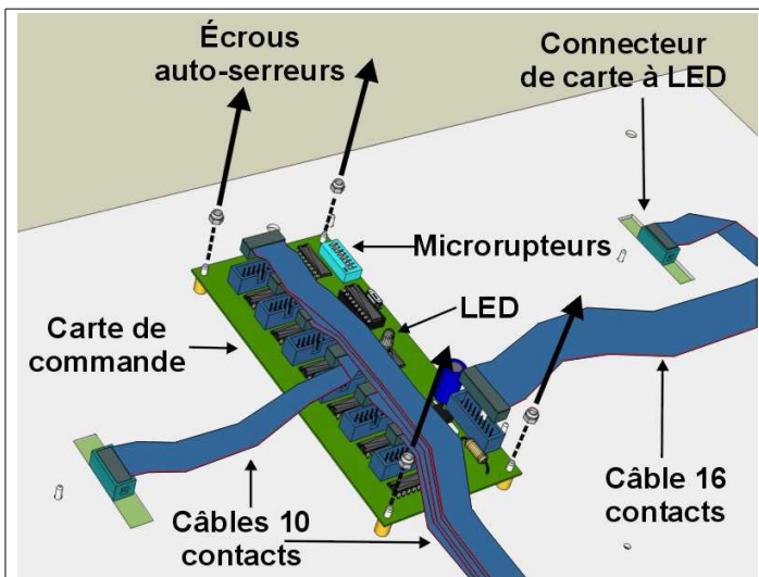
Fig. 19: Remplacement d'une carte de commande
