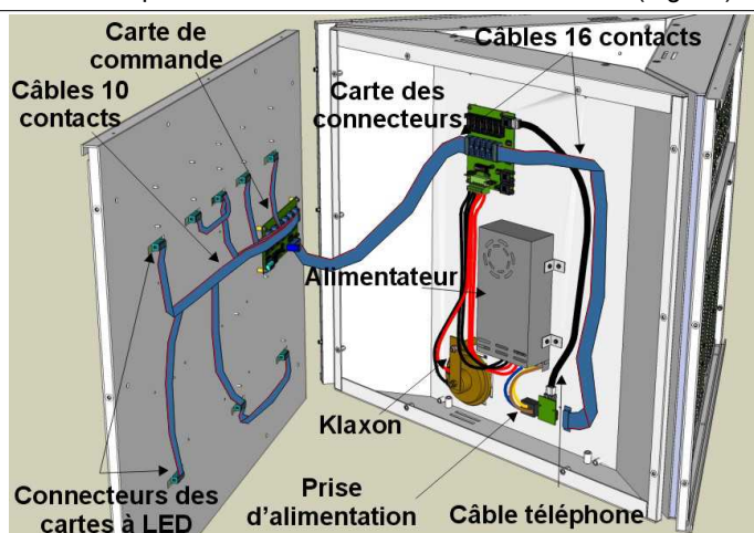
Fig. 18: Vue intérieure du module
