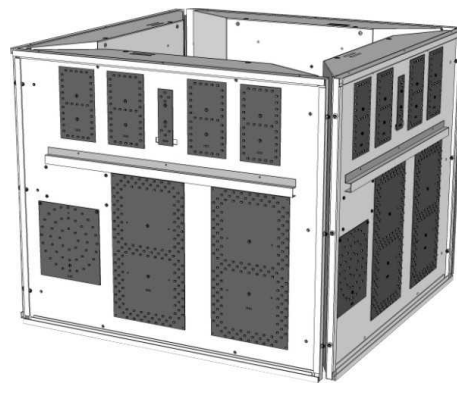
Fig. 3: FS-24s-4 (art.258-4) Affichage sur 4 faces
