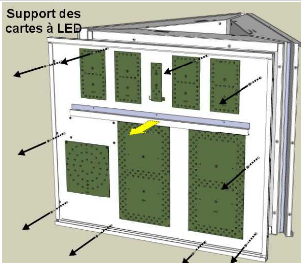
Fig. 17: Vis du support des cartes à LED
