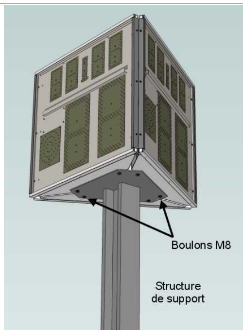
Fig. 9: Exemple de structure d'installation
