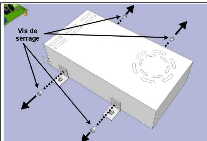
Fig. 22: Remplacement de l'alimentateur
