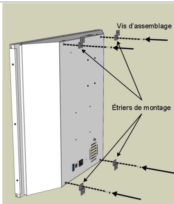
Fig. 10: Étriers de montage pour FS-24s-1
