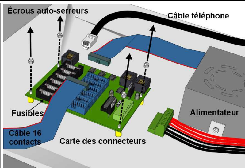
Fig. 21: Remplacement d'une carte des connecteurs
